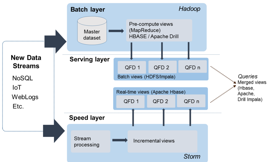
Figura 2. Composición detallada de la Arquitectura Lambda
